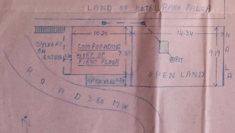
SITE PLAN SCALE 1:250
