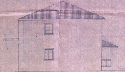
RIGHT ELEVATION
